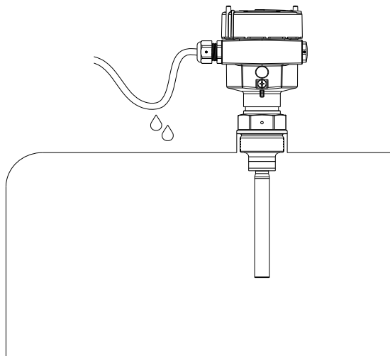
图 6 防潮安装
