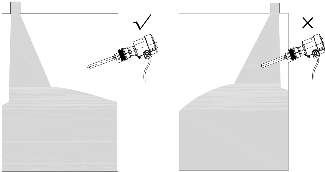
图 5 避开入料口的安装示意图
