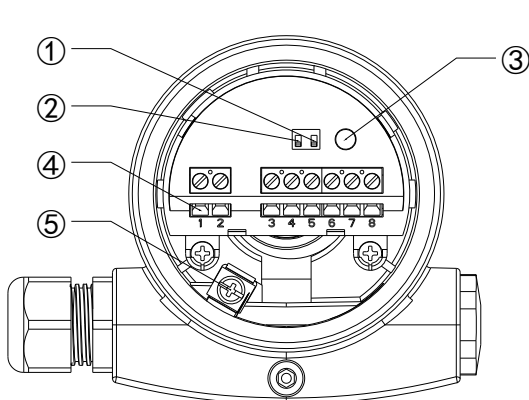
图 12 继电器输出方式
