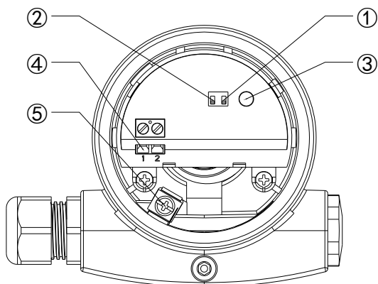
图 13 二线制输出方式
