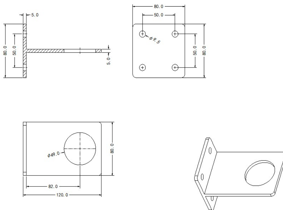
图 4 T 型支架示意图
